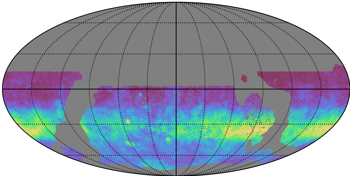
no_magell_roll_v3.4_10yrs WFD r band: AngleRms rotSkyPos
