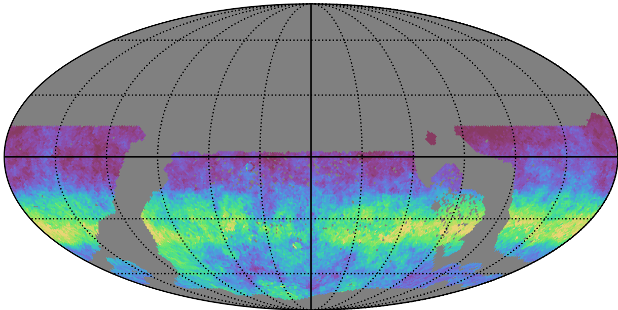
no_magell_roll_v3.4_10yrs WFD g band: AngleRms rotSkyPos
