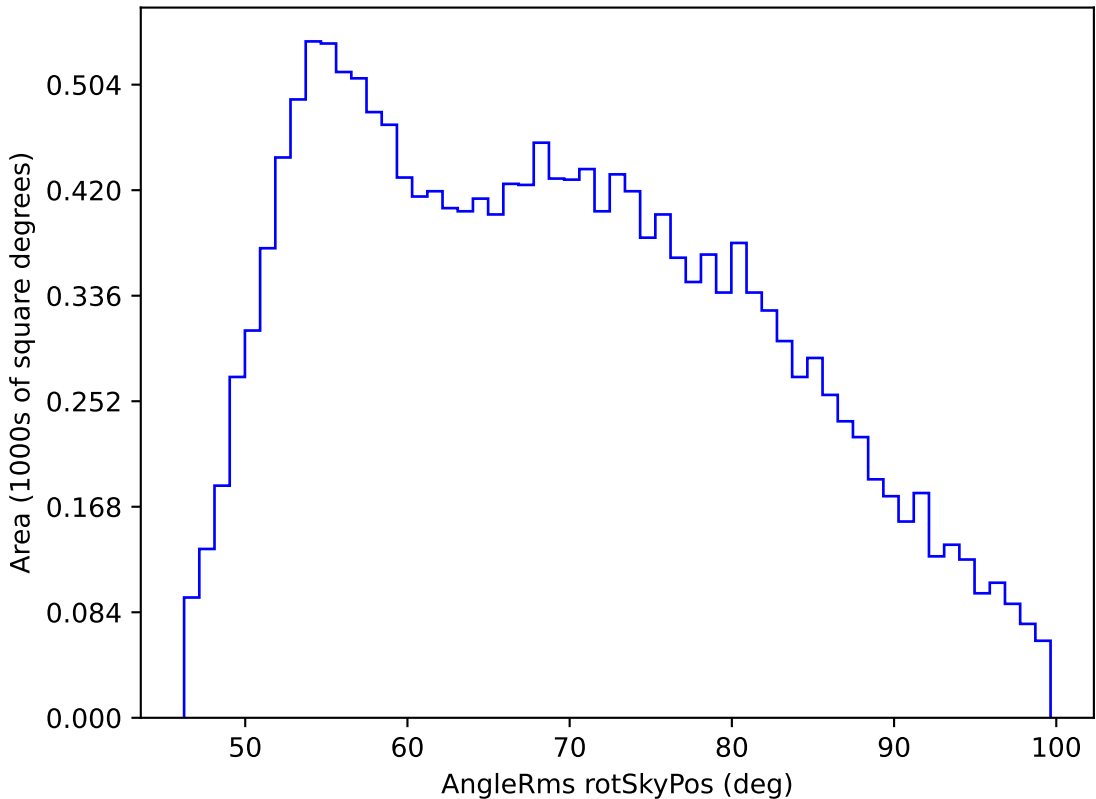
no_magell_roll_v3.4_10yrs WFD g band: AngleRms rotSkyPos
