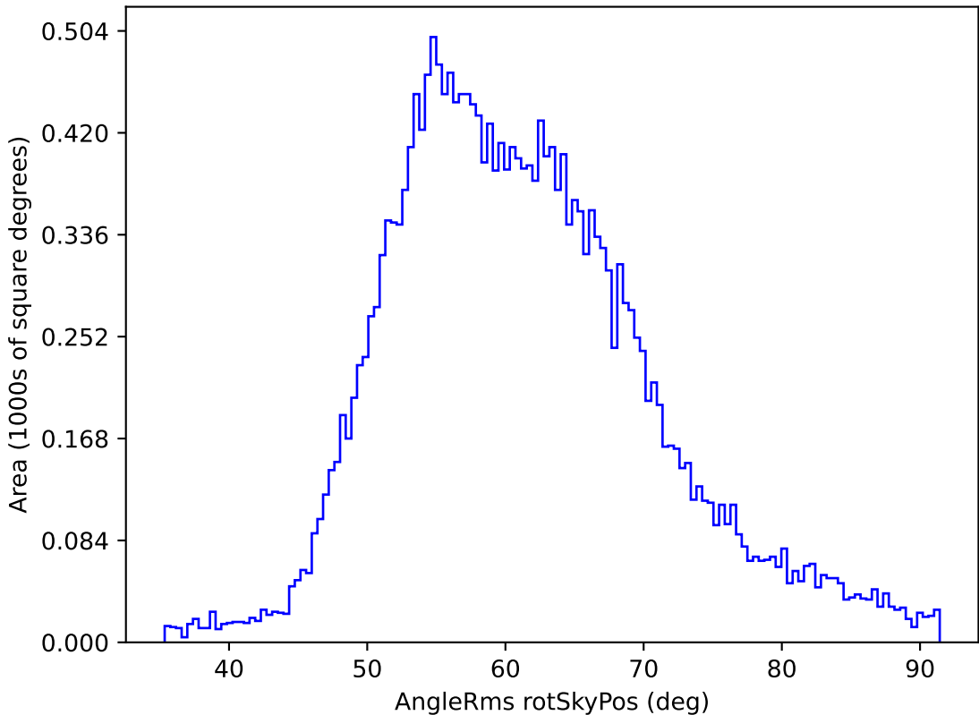
no_magell_roll_v3.4_10yrs All sky y band: AngleRms rotSkyPos
