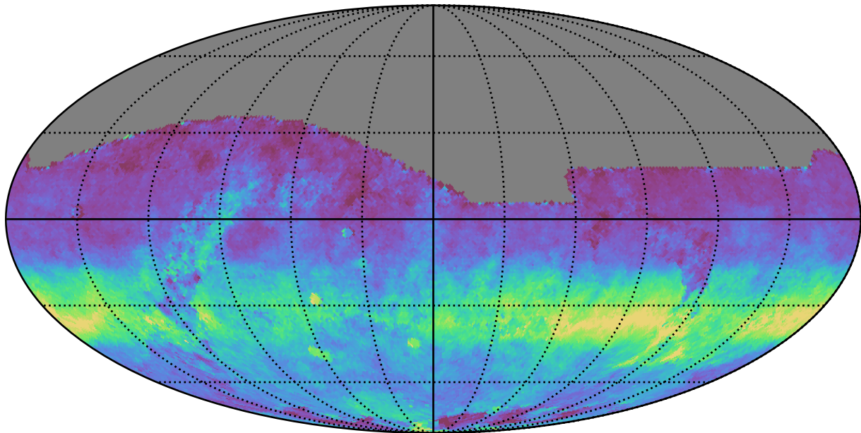
no_magell_roll_v3.4_10yrs All sky r band: AngleRms rotSkyPos
