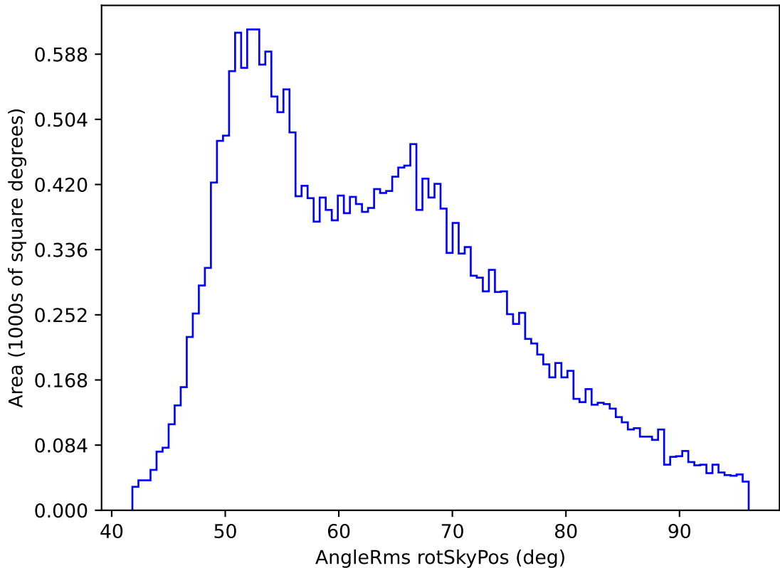
no_magell_roll_v3.4_10yrs All sky r band: AngleRms rotSkyPos
