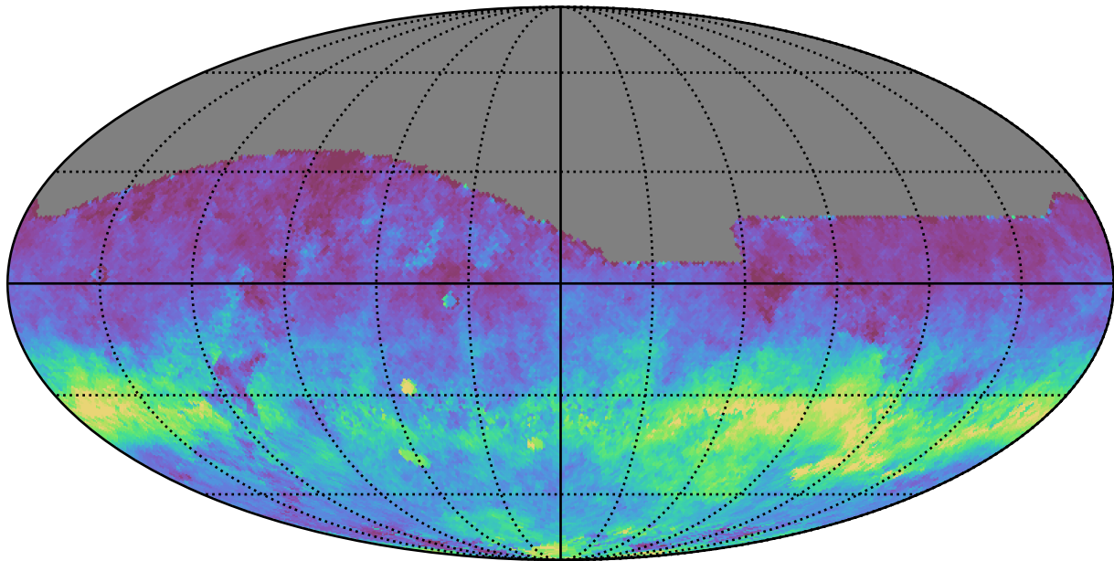
no_magell_roll_v3.4_10yrs All sky i band: AngleRms rotSkyPos
