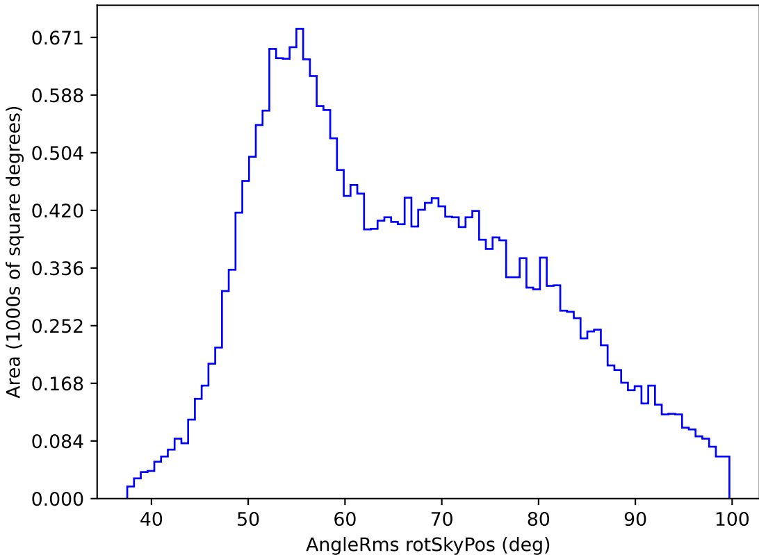
no_magell_roll_v3.4_10yrs All sky g band: AngleRms rotSkyPos
