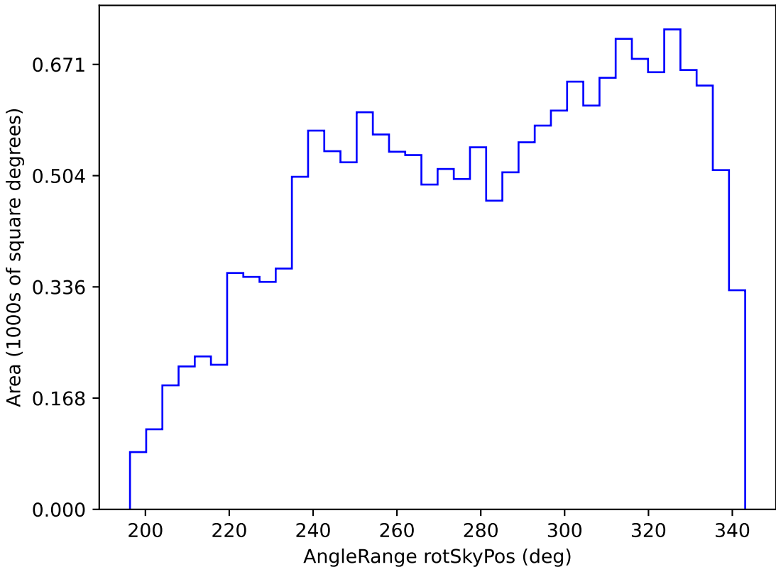
no_magell_roll_v3.4_10yrs WFD z band: AngleRange rotSkyPos
