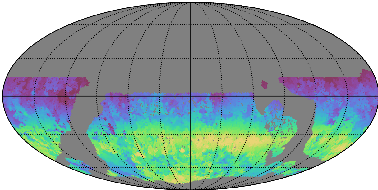
no_magell_roll_v3.4_10yrs WFD y band: AngleRange rotSkyPos
