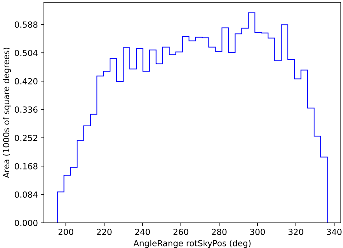
no_magell_roll_v3.4_10yrs WFD y band: AngleRange rotSkyPos
