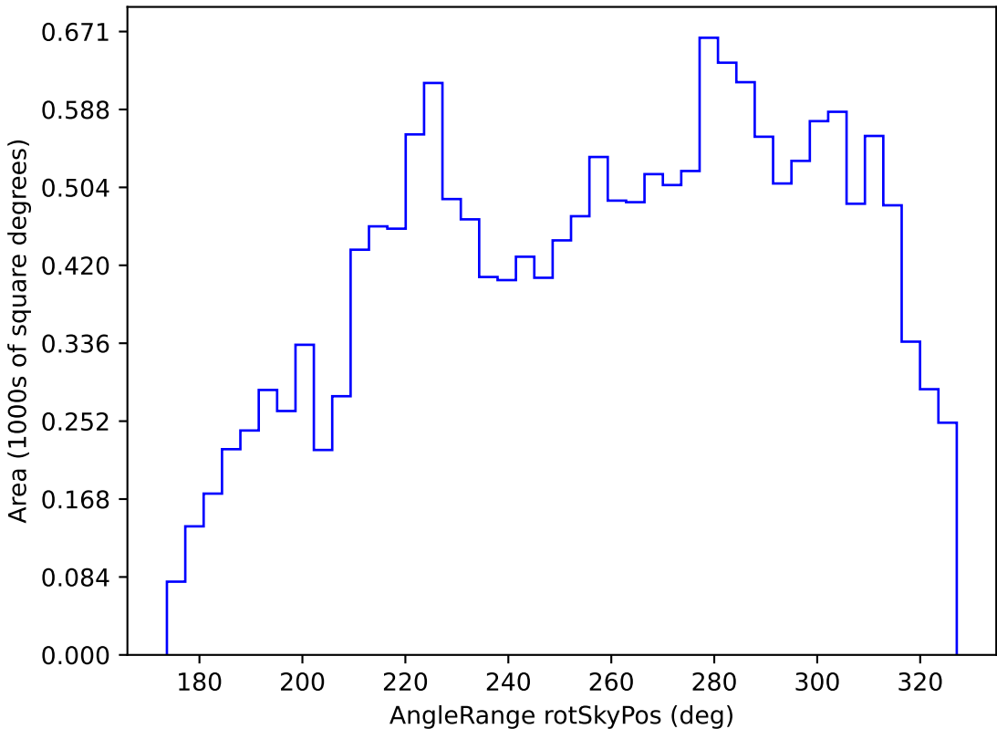
no_magell_roll_v3.4_10yrs WFD u band: AngleRange rotSkyPos
