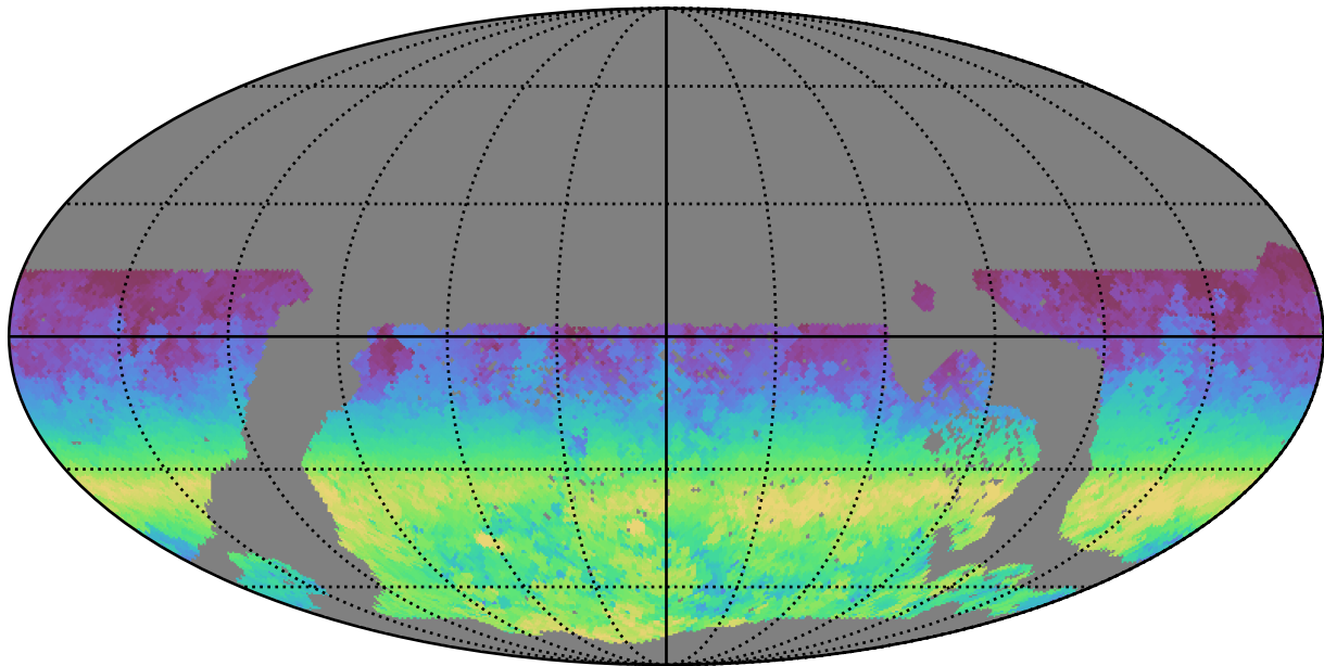
no_magell_roll_v3.4_10yrs WFD r band: AngleRange rotSkyPos
