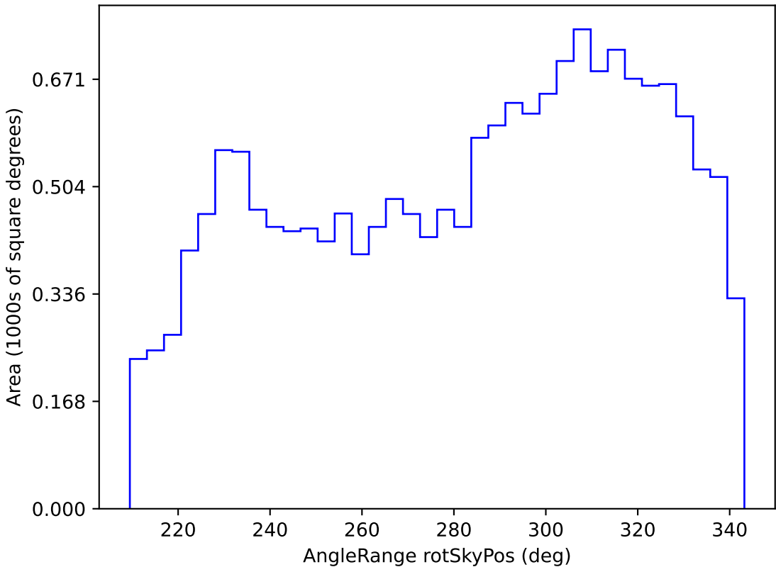
no_magell_roll_v3.4_10yrs WFD r band: AngleRange rotSkyPos
