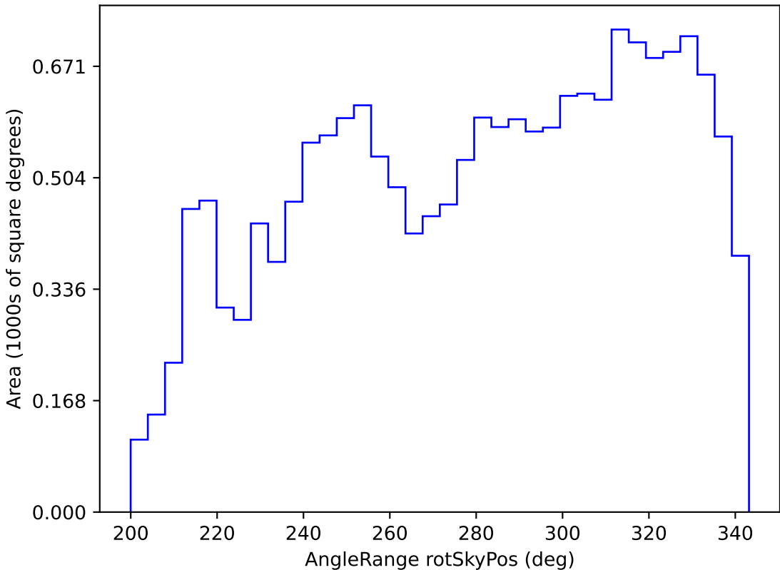
no_magell_roll_v3.4_10yrs WFD i band: AngleRange rotSkyPos
