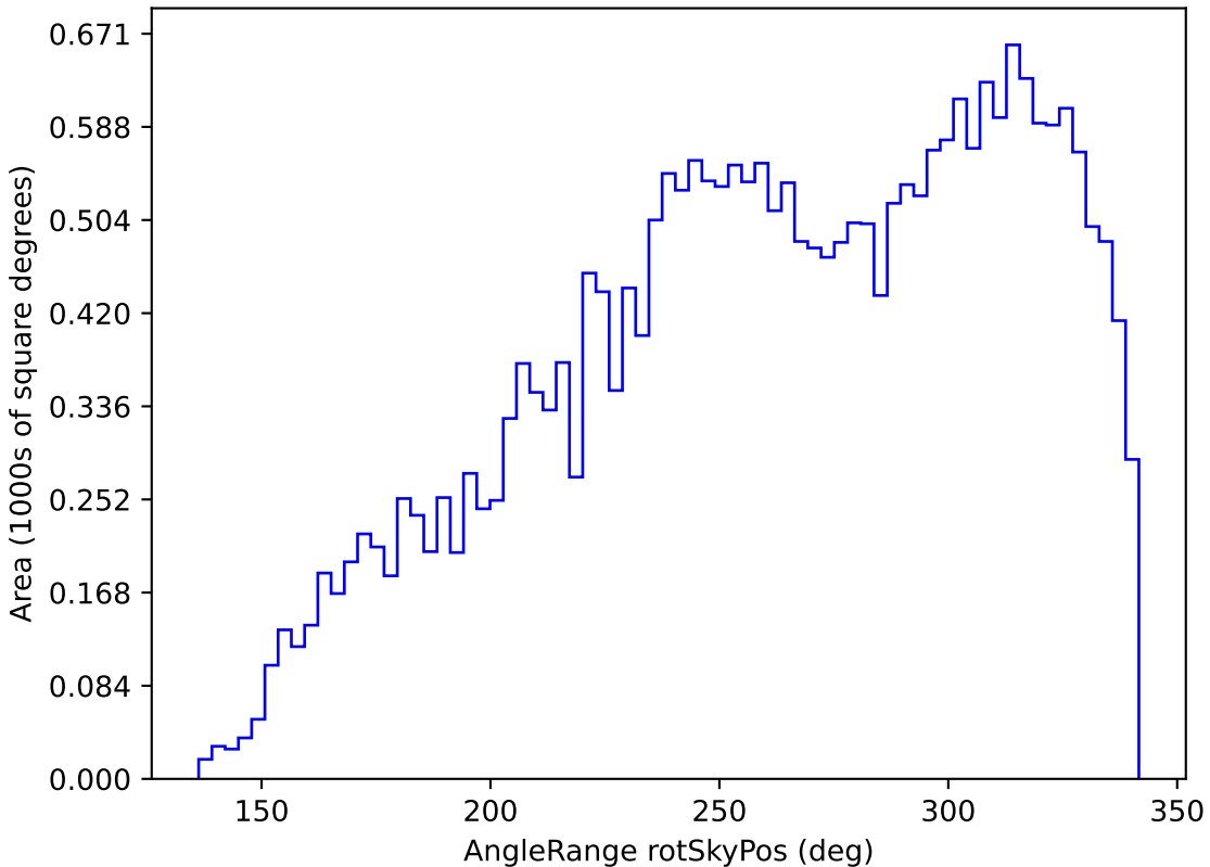
no_magell_roll_v3.4_10yrs All sky z band: AngleRange rotSkyPos
