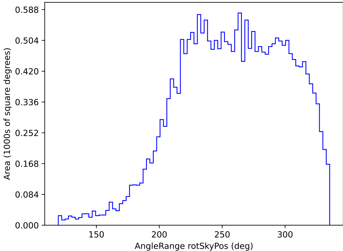
no_magell_roll_v3.4_10yrs All sky y band: AngleRange rotSkyPos
