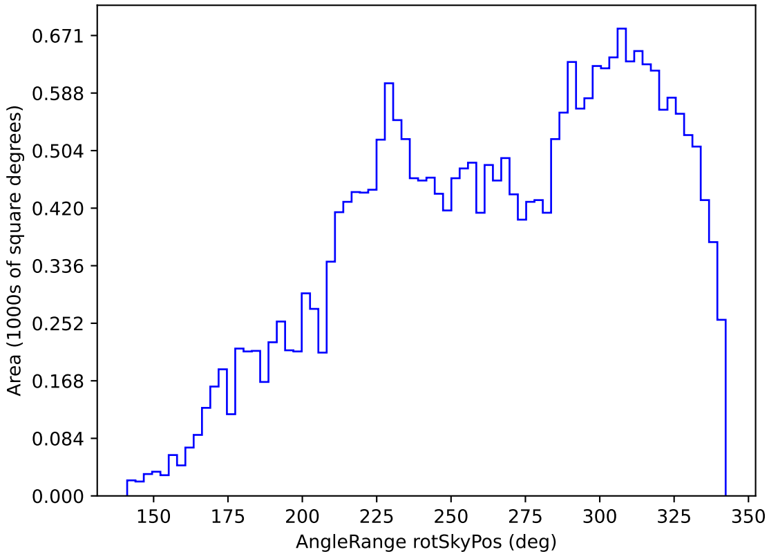
no_magell_roll_v3.4_10yrs All sky r band: AngleRange rotSkyPos
