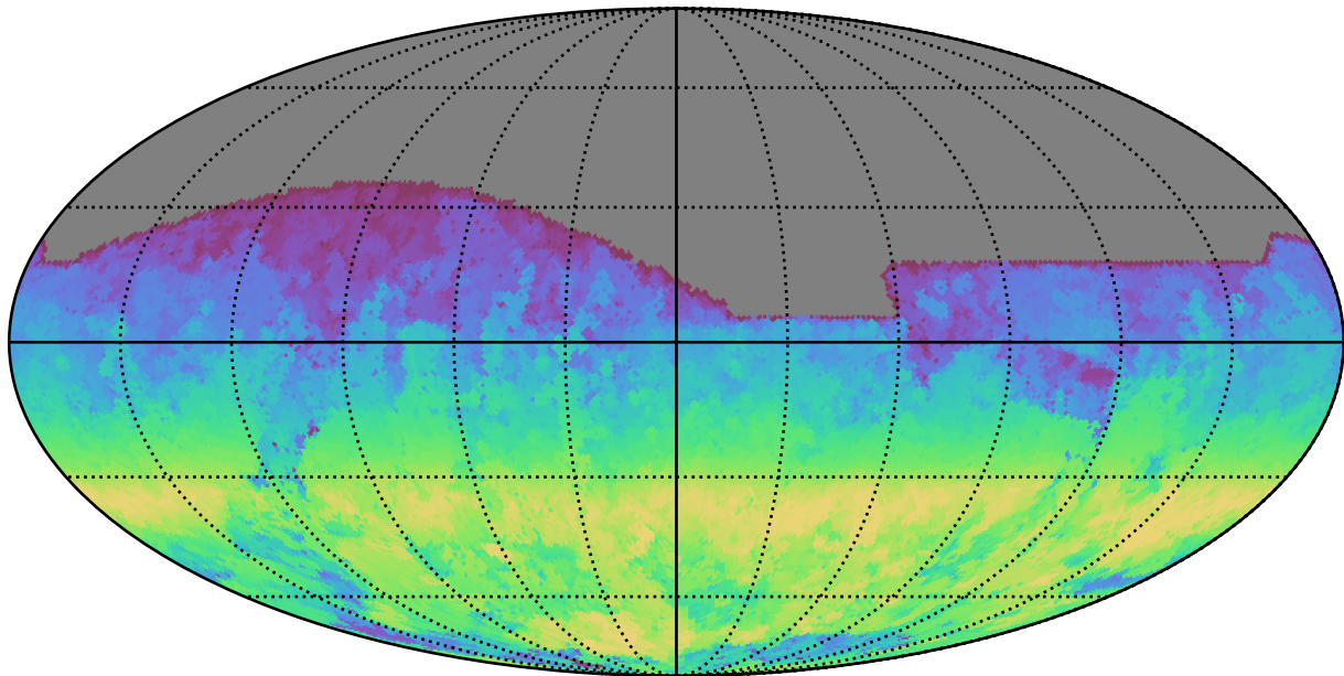
no_magell_roll_v3.4_10yrs All sky i band: AngleRange rotSkyPos
