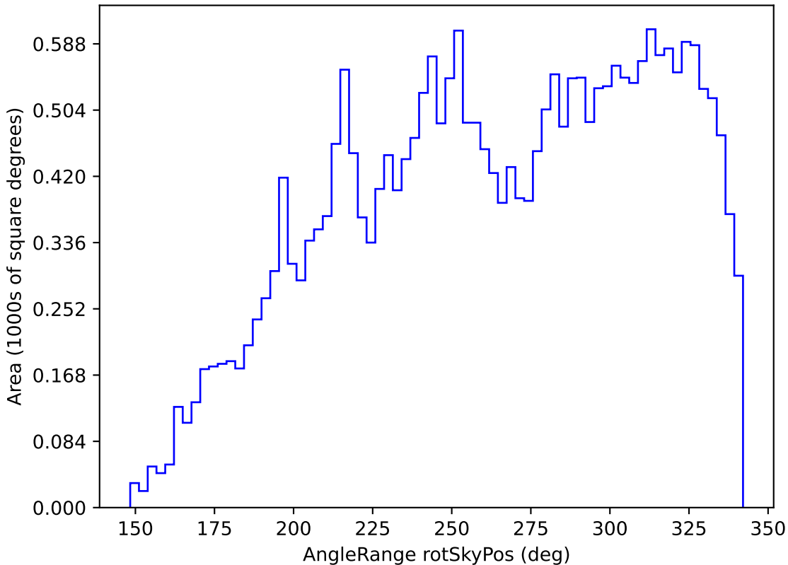
no_magell_roll_v3.4_10yrs All sky i band: AngleRange rotSkyPos
