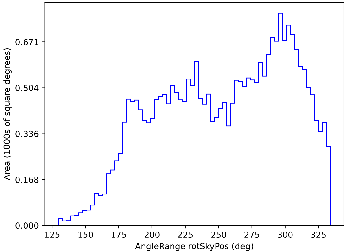
no_magell_roll_v3.4_10yrs All sky g band: AngleRange rotSkyPos
