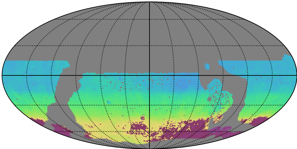
no_magell_roll_v3.4_10yrs WFD z band: AngleMean rotSkyPos
