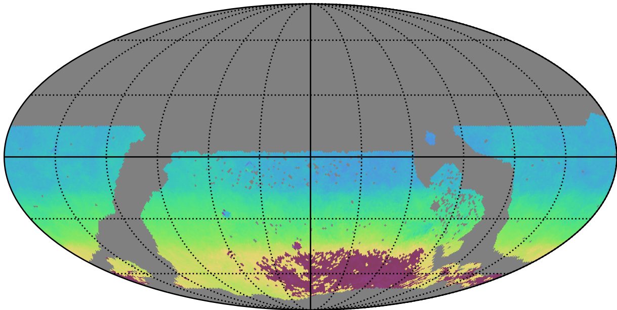
no_magell_roll_v3.4_10yrs WFD y band: AngleMean rotSkyPos
