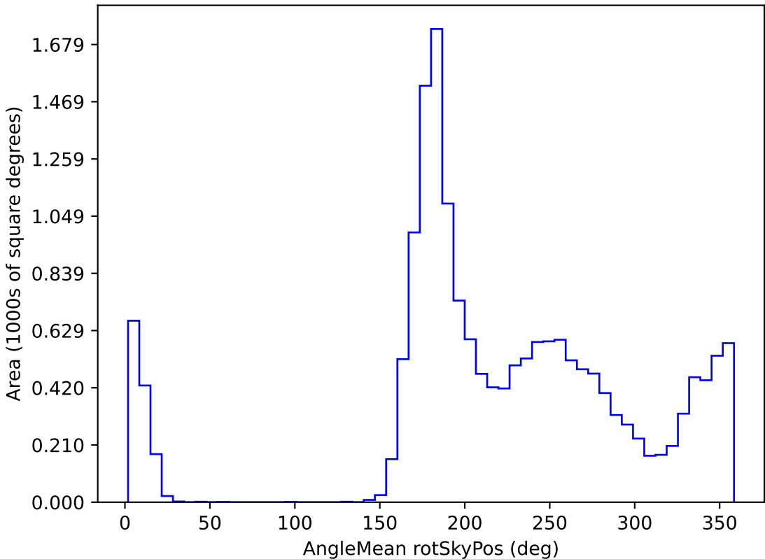
no_magell_roll_v3.4_10yrs WFD y band: AngleMean rotSkyPos
