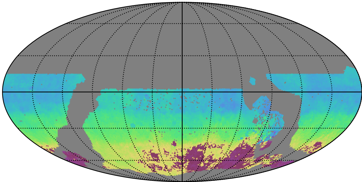
no_magell_roll_v3.4_10yrs WFD u band: AngleMean rotSkyPos
