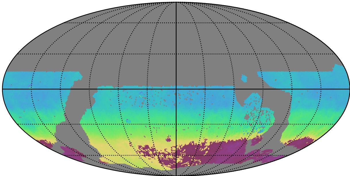
no_magell_roll_v3.4_10yrs WFD r band: AngleMean rotSkyPos
