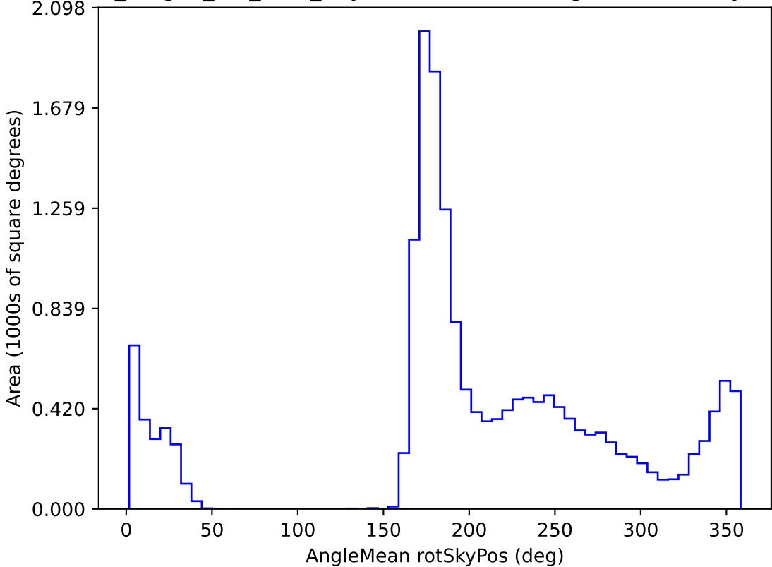
no_magell_roll_v3.4_10yrs WFD r band: AngleMean rotSkyPos
