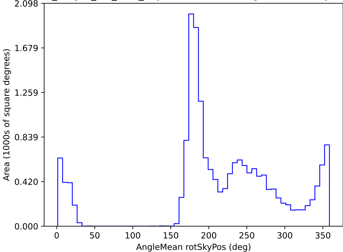
no_magell_roll_v3.4_10yrs WFD i band: AngleMean rotSkyPos
