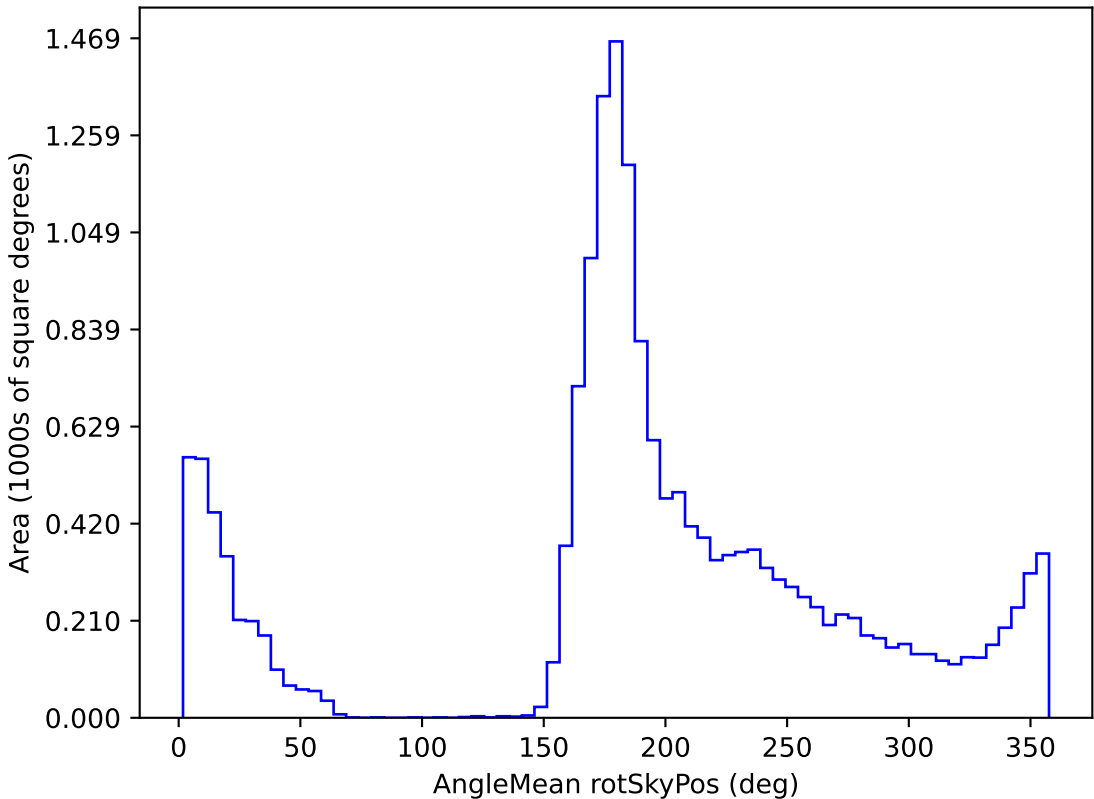
no_magell_roll_v3.4_10yrs WFD g band: AngleMean rotSkyPos
