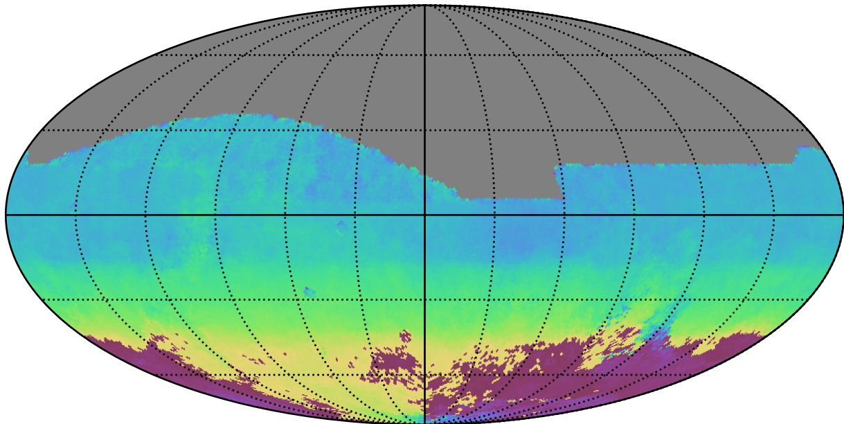
no_magell_roll_v3.4_10yrs All sky z band: AngleMean rotSkyPos
