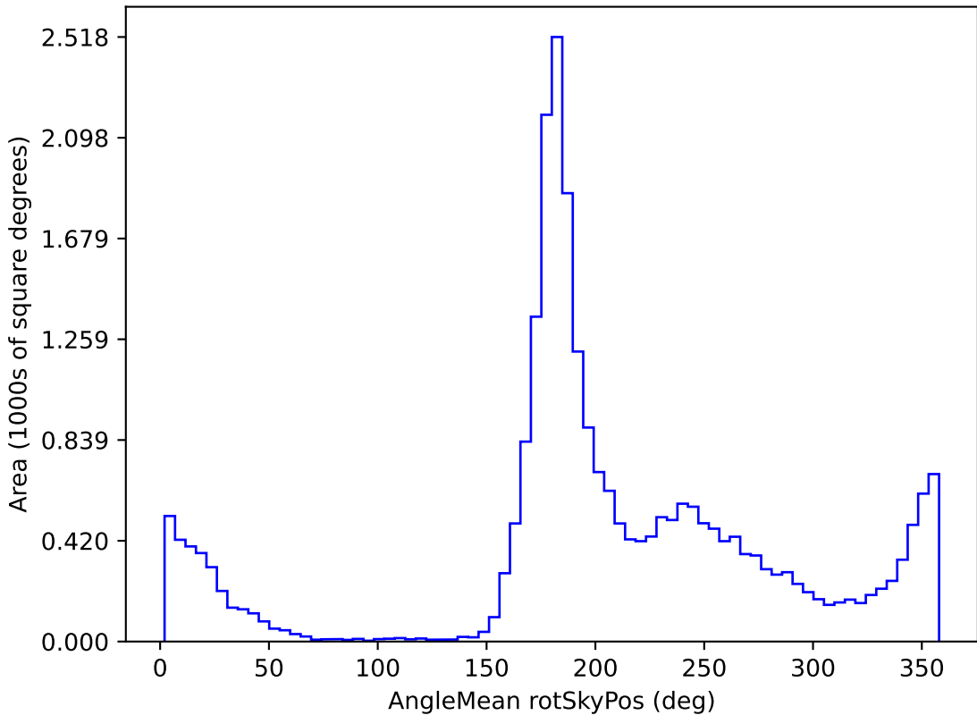
no_magell_roll_v3.4_10yrs All sky z band: AngleMean rotSkyPos
