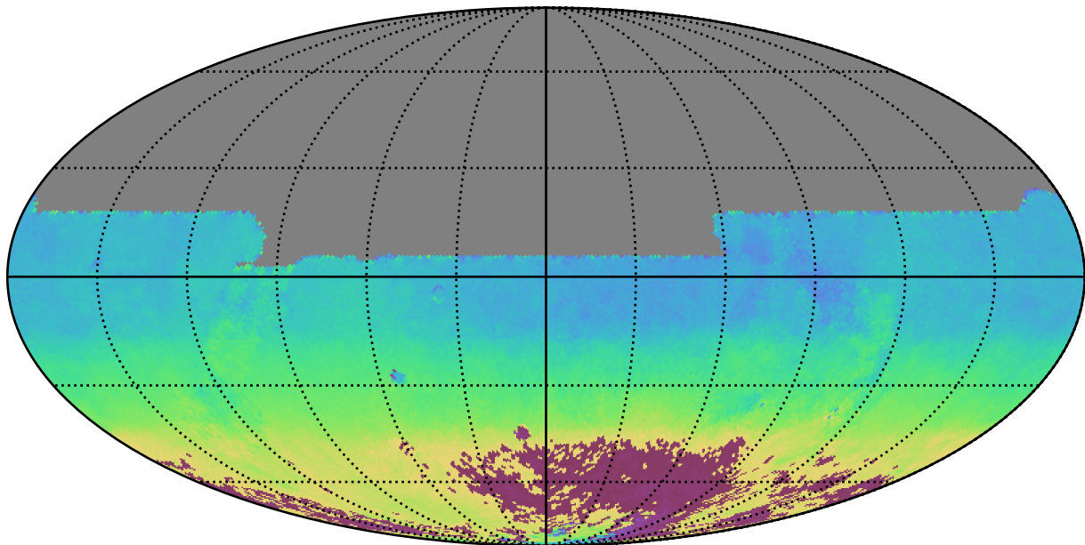
no_magell_roll_v3.4_10yrs All sky y band: AngleMean rotSkyPos
