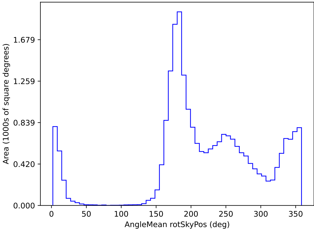
no_magell_roll_v3.4_10yrs All sky y band: AngleMean rotSkyPos
