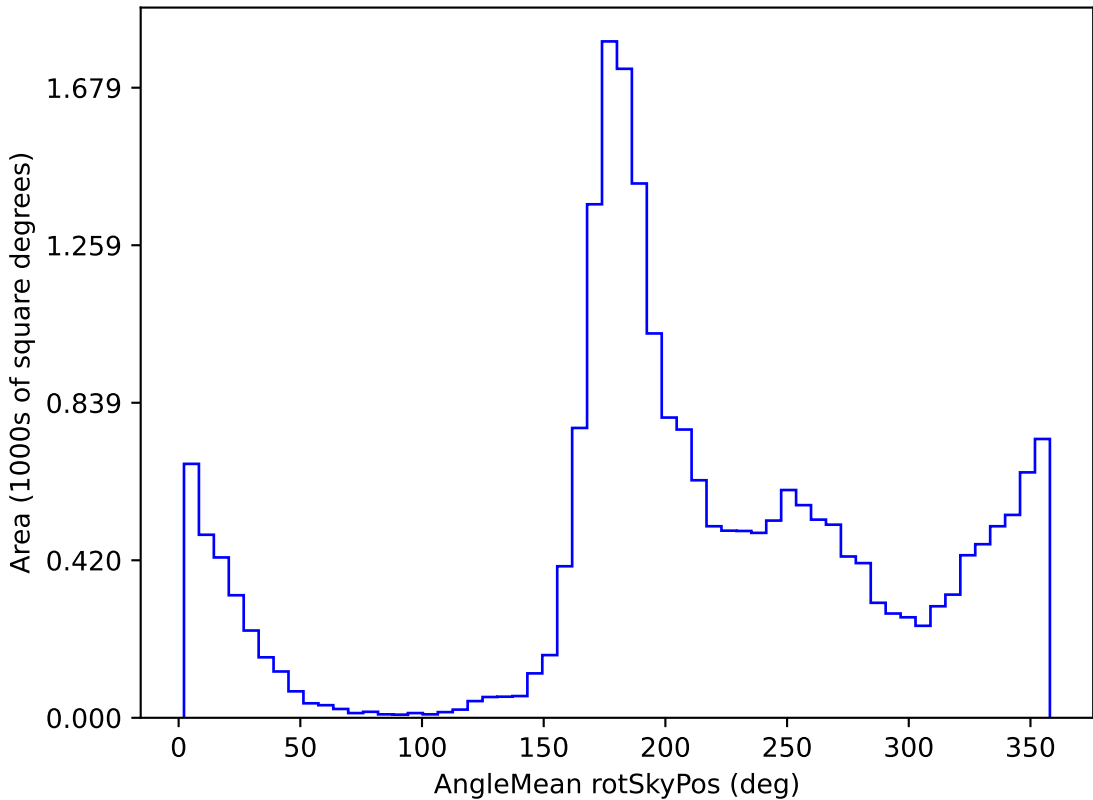
no_magell_roll_v3.4_10yrs All sky u band: AngleMean rotSkyPos
