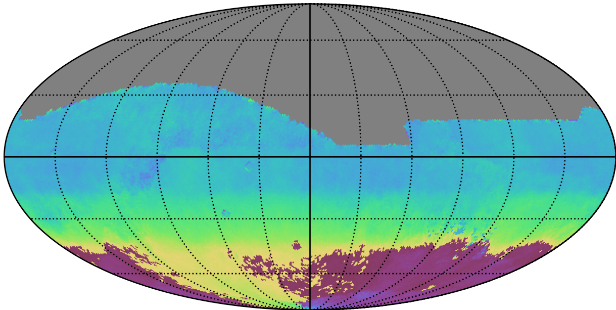
no_magell_roll_v3.4_10yrs All sky r band: AngleMean rotSkyPos
