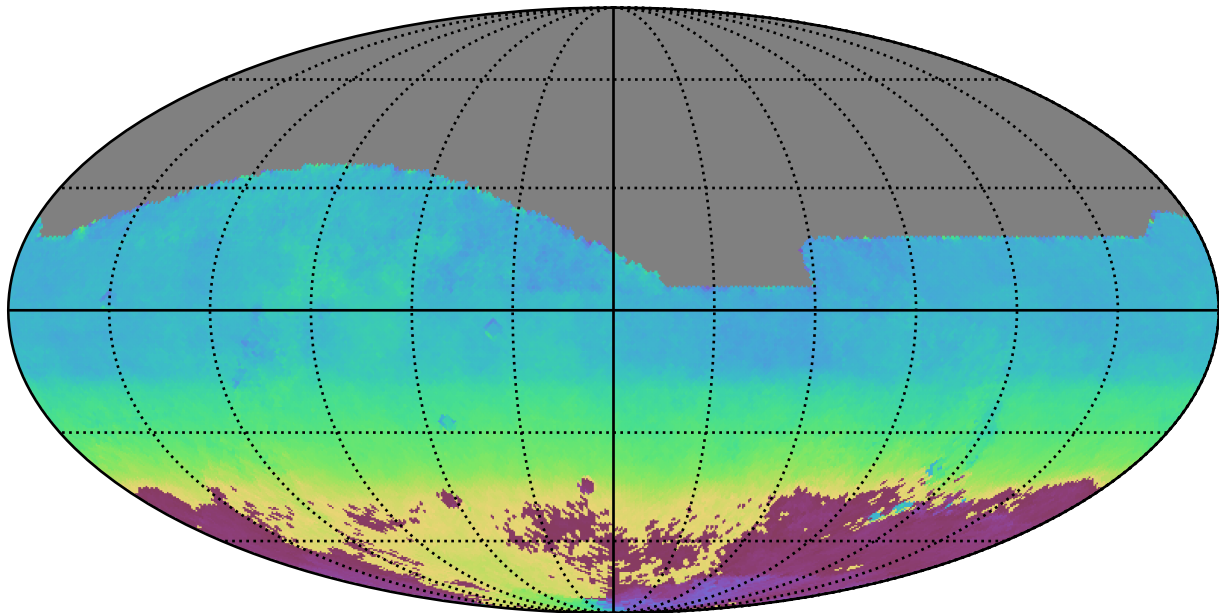
no_magell_roll_v3.4_10yrs All sky i band: AngleMean rotSkyPos
