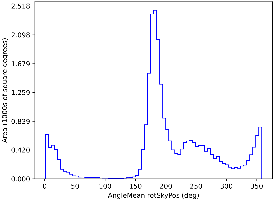
no_magell_roll_v3.4_10yrs All sky i band: AngleMean rotSkyPos
