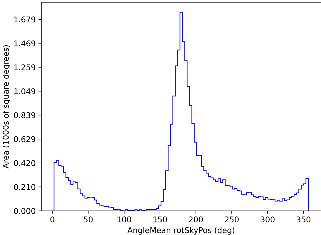
no_magell_roll_v3.4_10yrs All sky g band: AngleMean rotSkyPos
