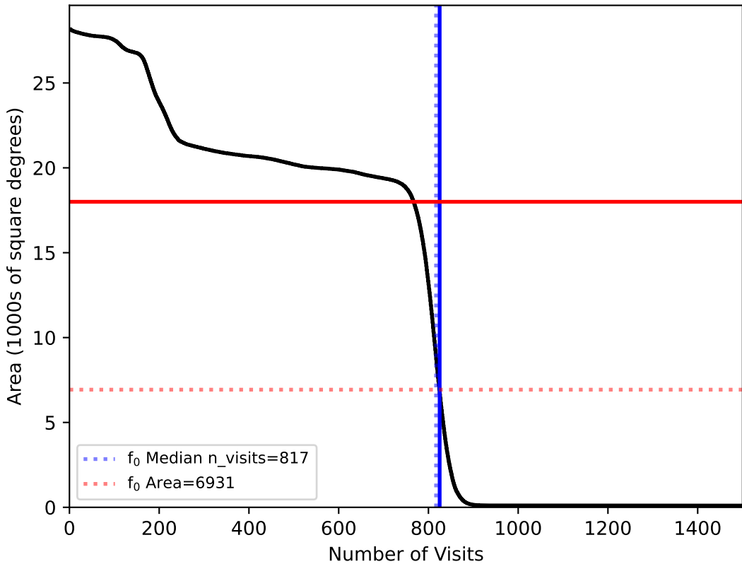
no_magell_roll_v3.4_10yrs : f0
