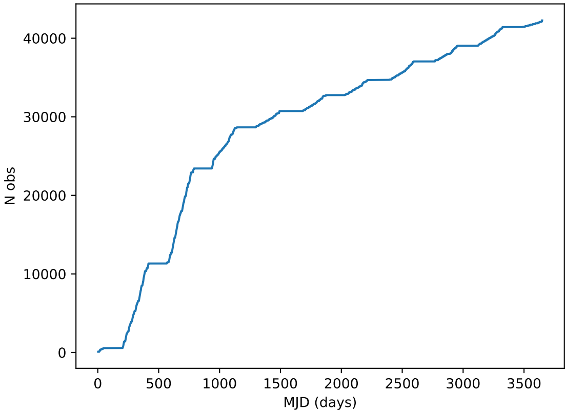
no_magell_roll_v3.4_10yrs note like DD:COSMOS%: Cumulative
