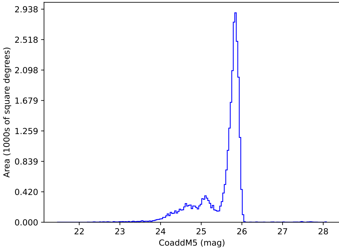
no_magell_roll_v3.4_10yrs z: CoaddM5
