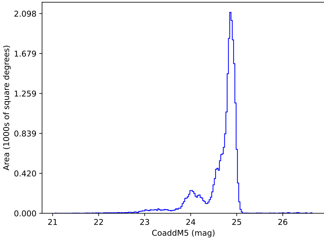
no_magell_roll_v3.4_10yrs y: CoaddM5
