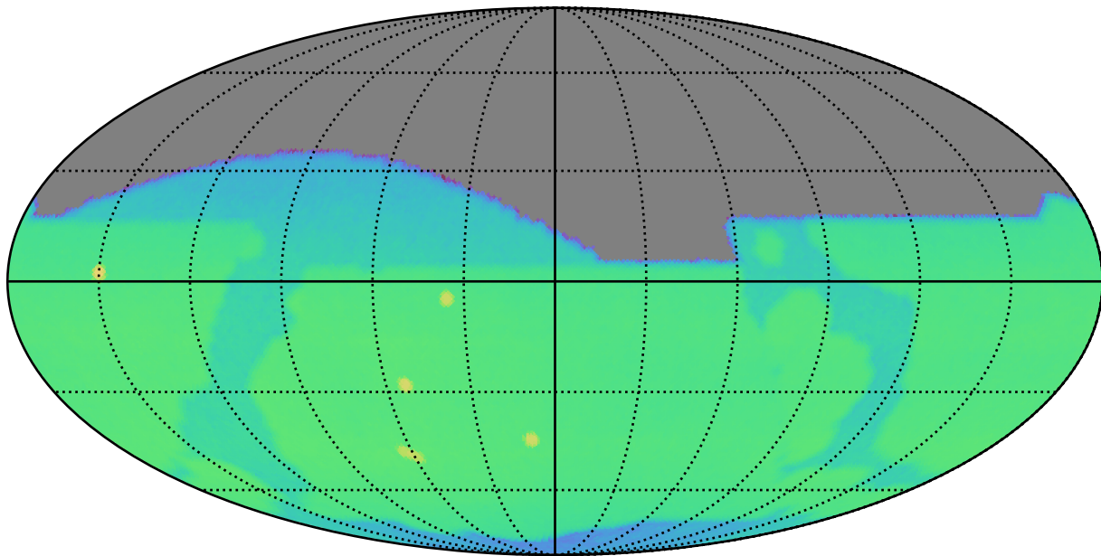
no_magell_roll_v3.4_10yrs r: CoaddM5
