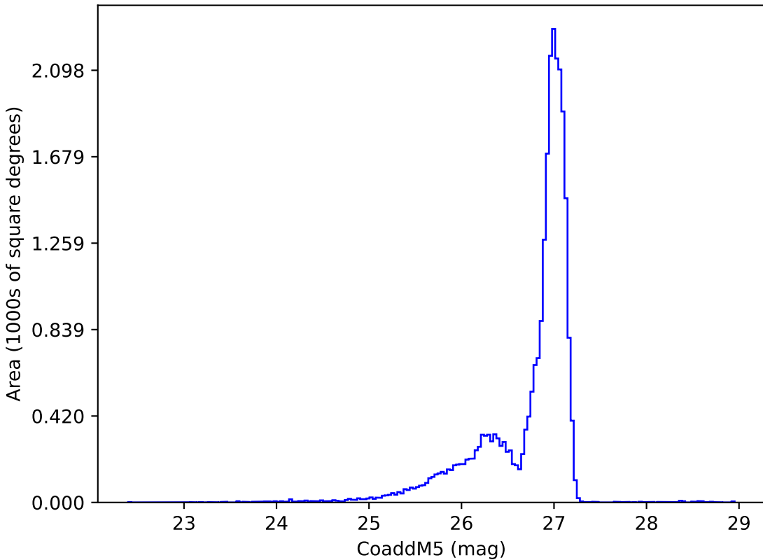
no_magell_roll_v3.4_10yrs r: CoaddM5
