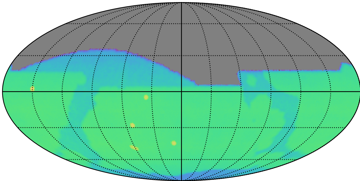
no_magell_roll_v3.4_10yrs i: CoaddM5
