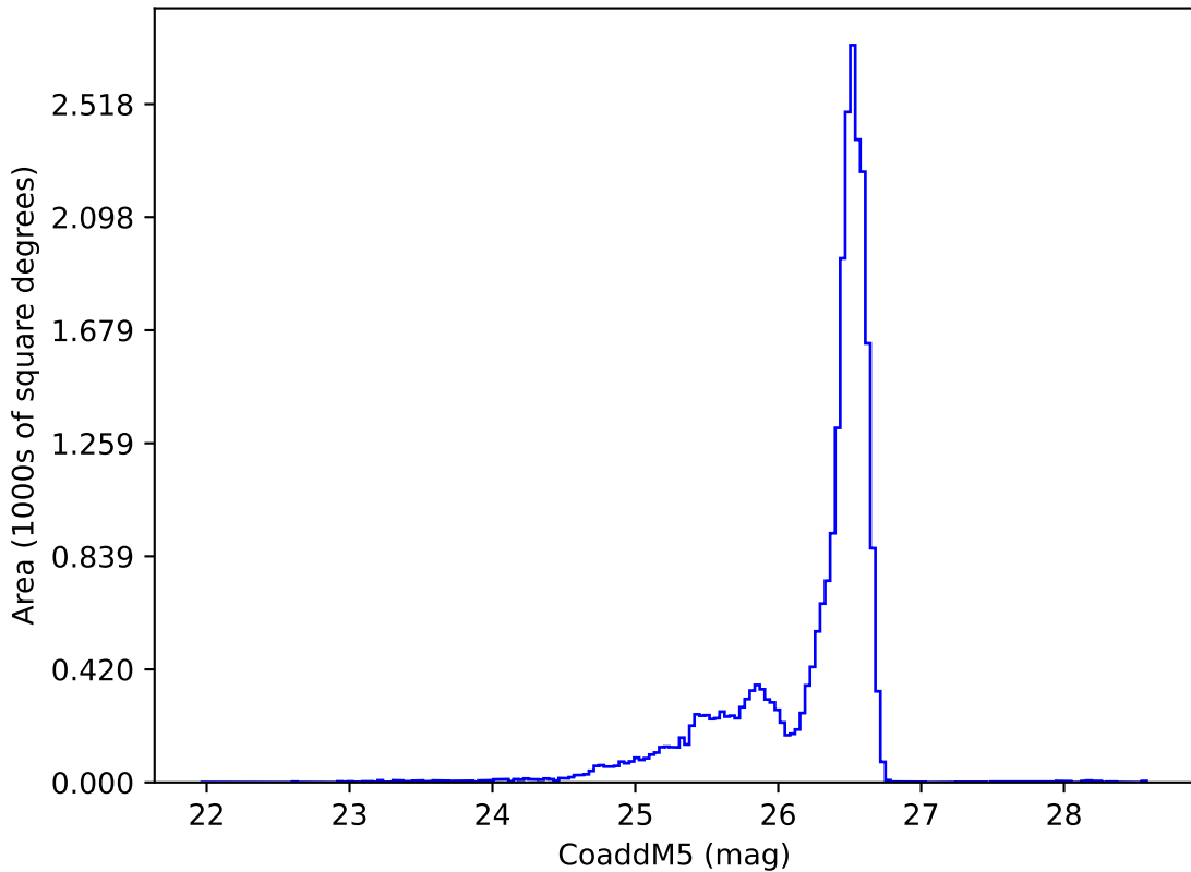
no_magell_roll_v3.4_10yrs i: CoaddM5
