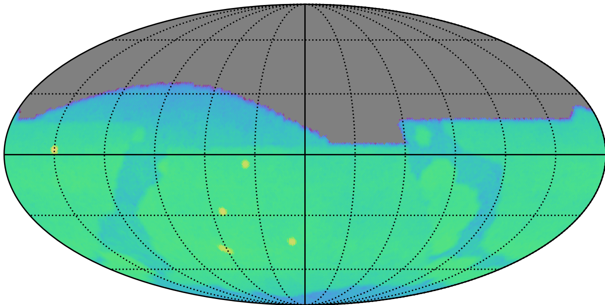
no_magell_roll_v3.4_10yrs g: CoaddM5
