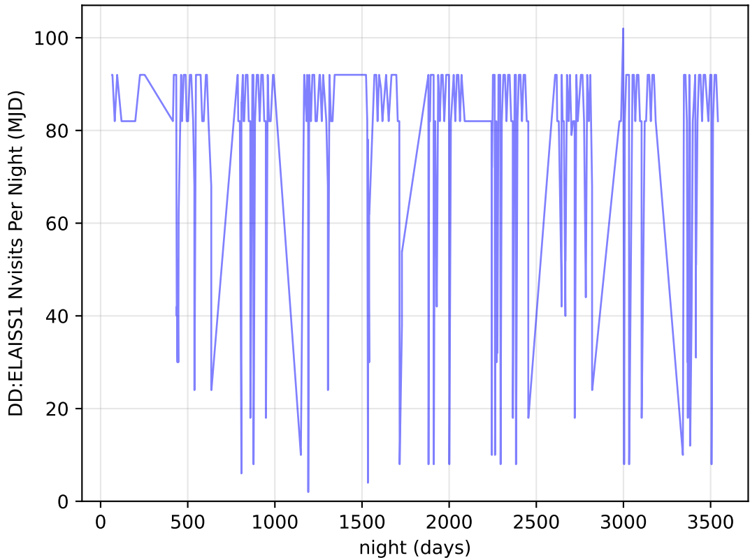
no_magell_roll_v3.4_10yrs all bands: DD:ELAISS1 Nvisits Per Night
