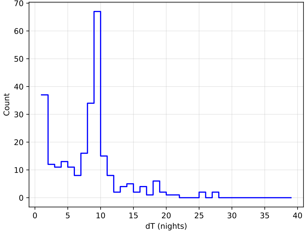
no_magell_roll_v3.4_10yrs all bands: DD:ELAISS1 Delta Nights Histogram
