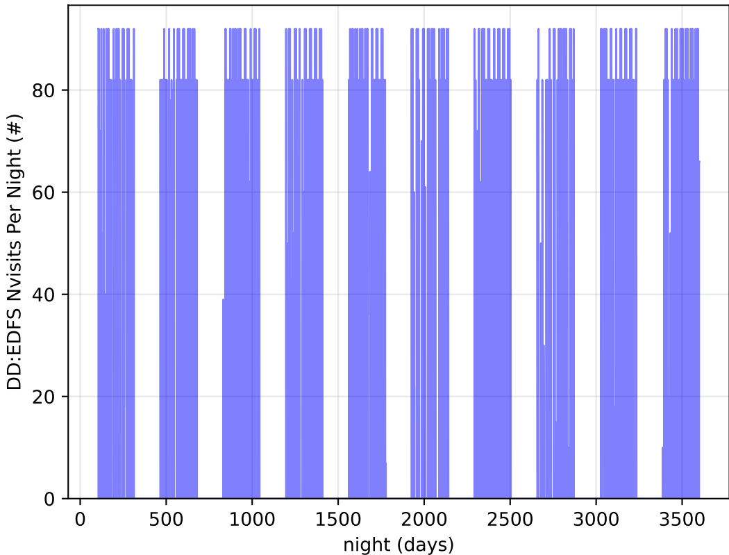
no_magell_roll_v3.4_10yrs all bands: DD:EDFS Nvisits Per Night
